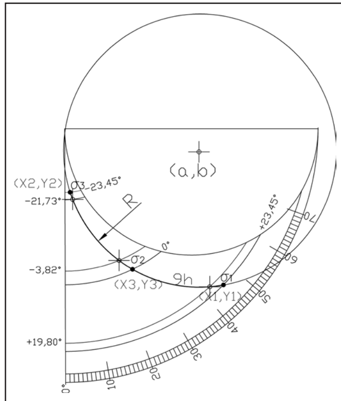
Fig. 3: Cirkel door drie punten van de 9h zonnetijdcurve
