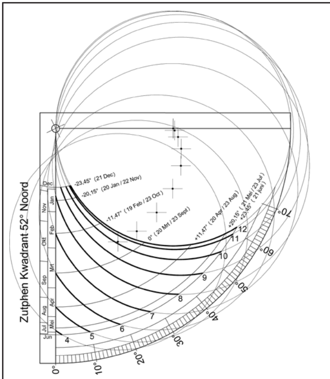
Fig. 4: Zonnetijdcurven 12h-4h vervangen door cirkelboog
