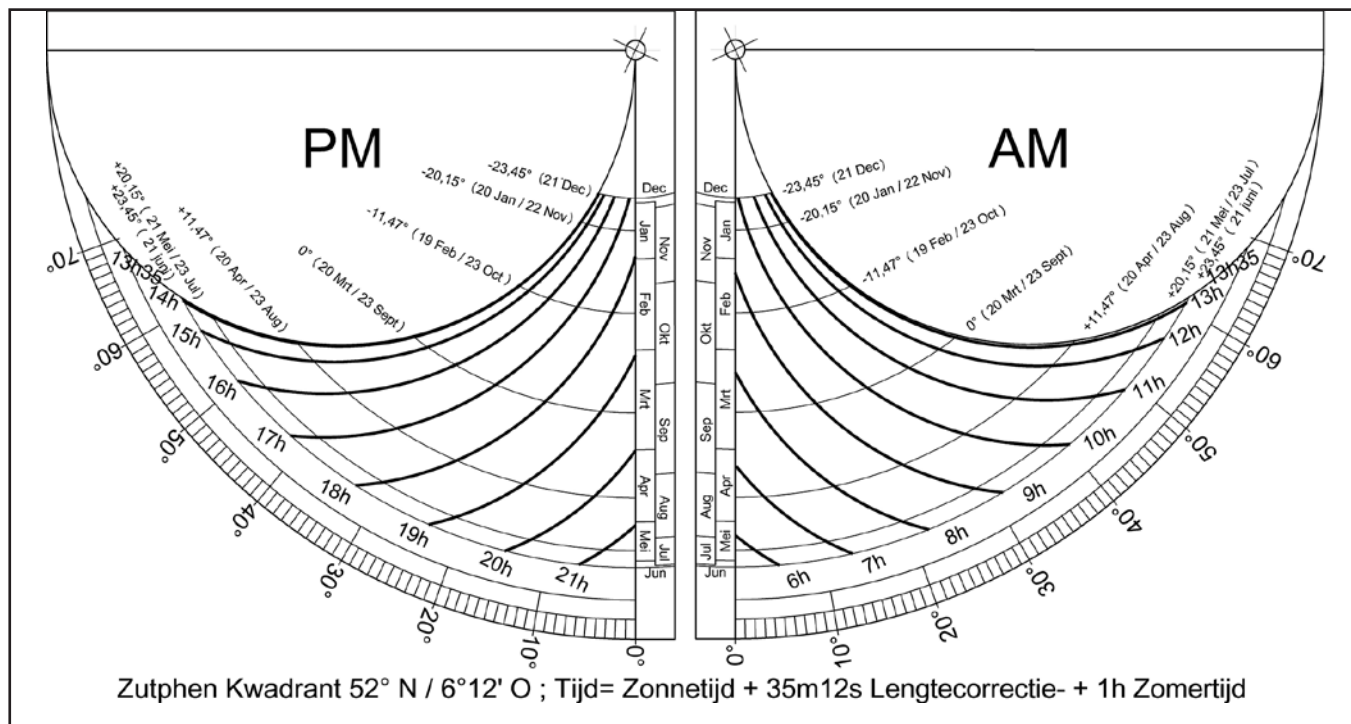
Fig.5: Kwadrant met gecorrigeerde zonnetijdcurven.
