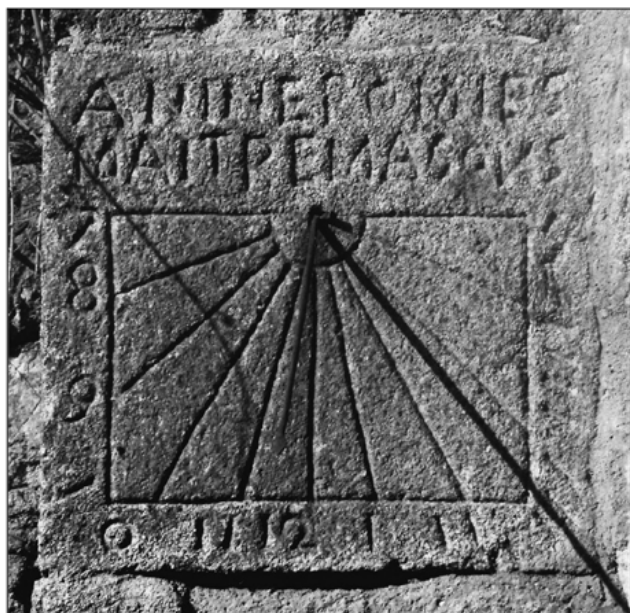
Fig. 7. De muurzonnewijzer in La Séauve-sur-Semène. Bron: [8].
