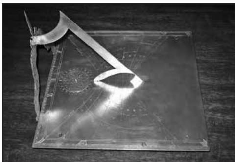
Een kijkje op de zorgvuldig gerestaureerde zonnewijzer van het kasteel de Renaissance te Oostmalle.
